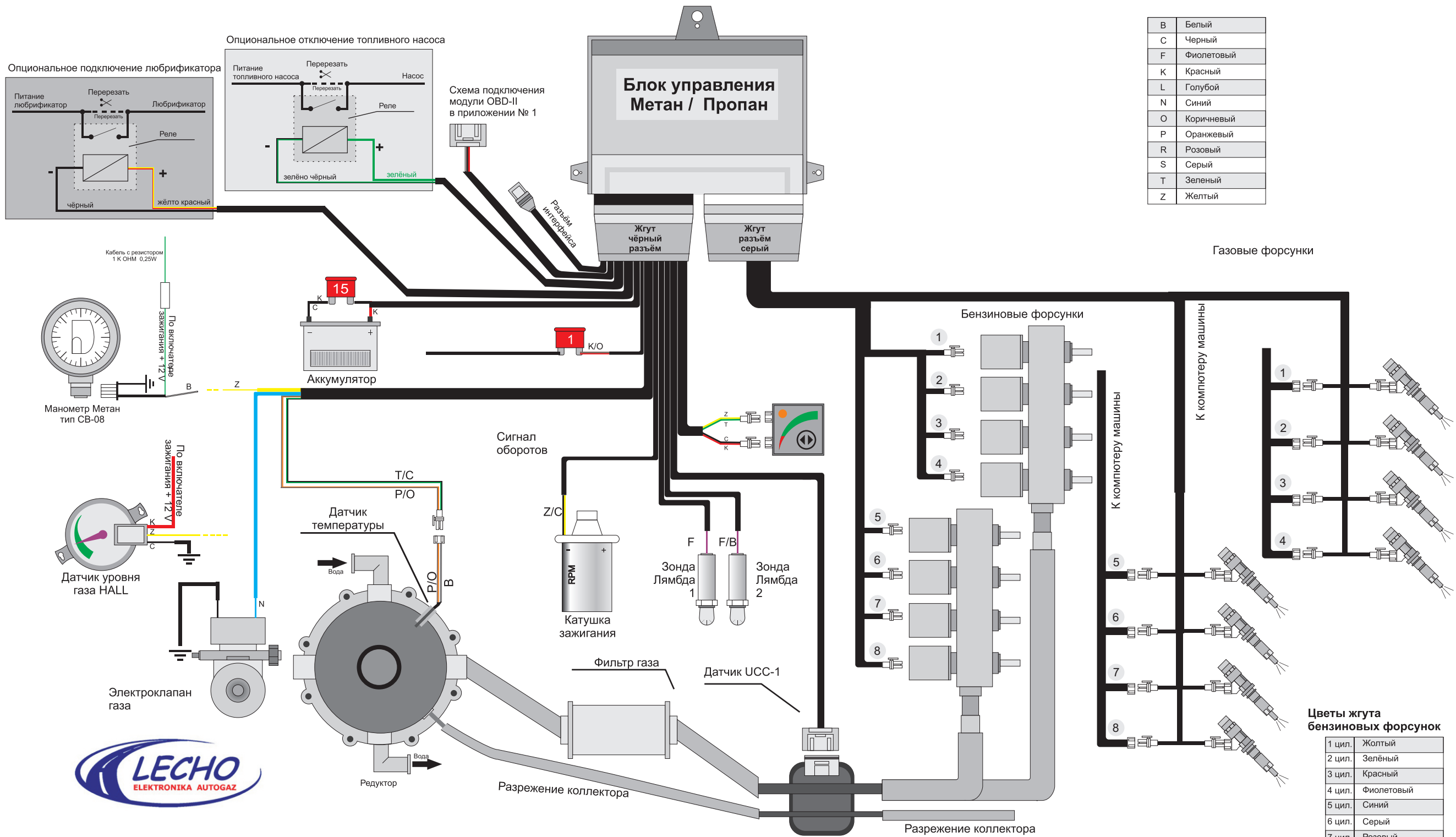
Схема подключения
